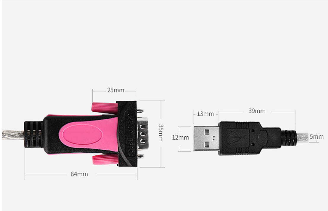
线缆尺寸图
